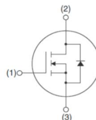
TO-247-3L
